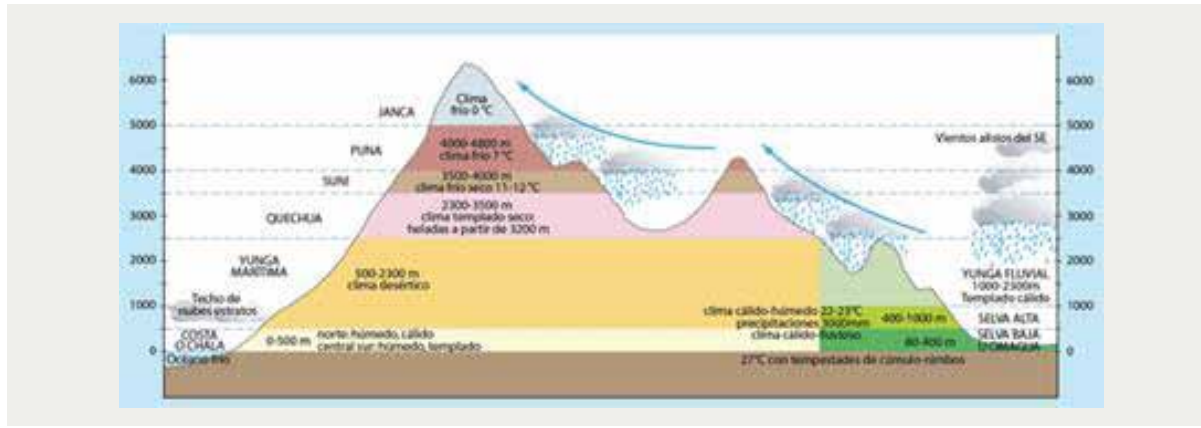
FIGURA 2.2. Perfil orográfico tipo del Perú
